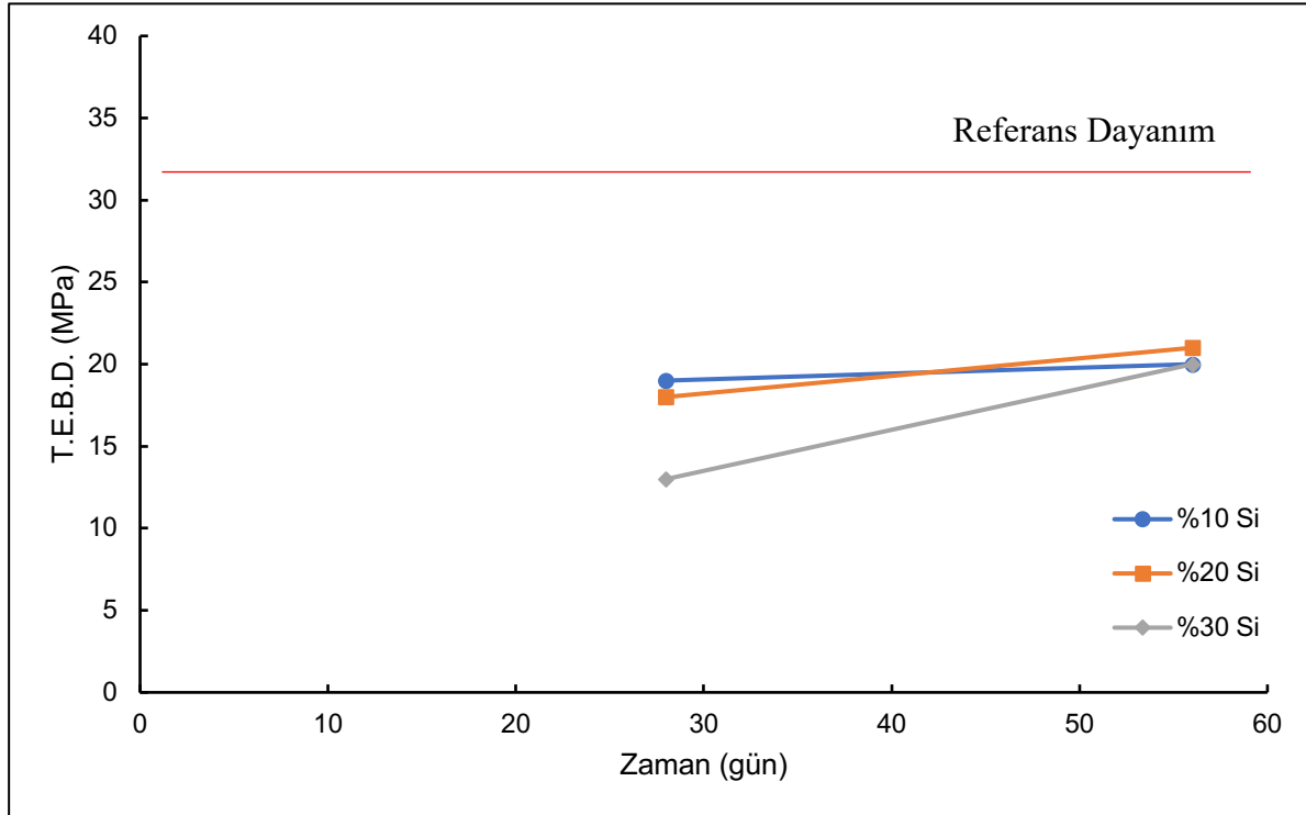
Şekil 4. %10-20-30 ikame oranlarındaki 28-56 günlük kür sürelerine göre dayanım değerleri
