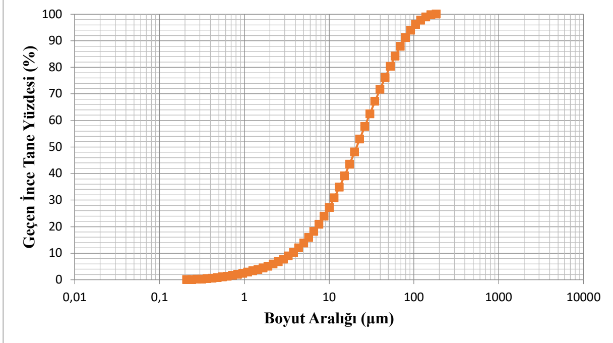
Şekil 1. Silis ocağı proses atığı tane boyut dağılımı
