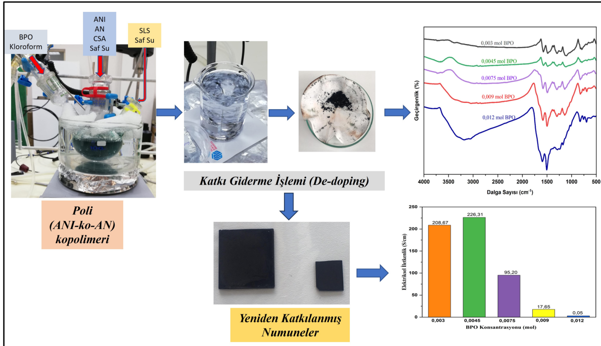
Şekil 1. Polimerizasyon ve devamında cam üzerine kaplanmış poli(ANI-ko-AN) kopolimer ince filmlerin eldesi için yapılan işlemler.
