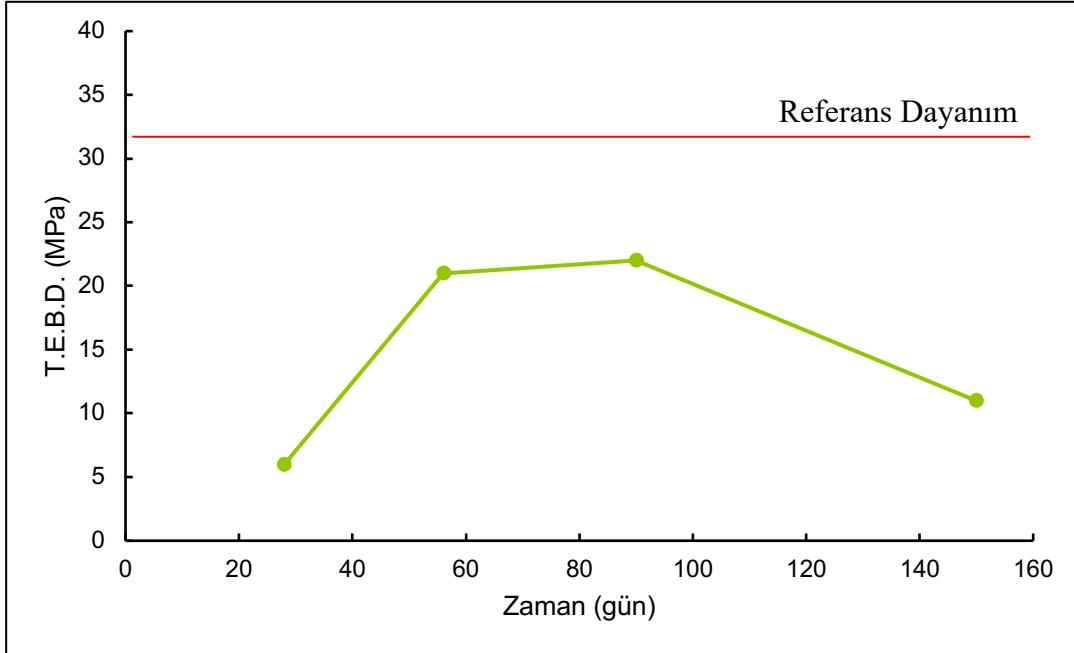
Şekil 4: %20 Altın madeni proses atığı ikamesinde zamana göre dayanım değerleri
