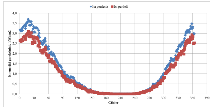
Şekil 2. Kırşehir ili iklim koşullarında günlük ısı enerjisi gereksinimi
