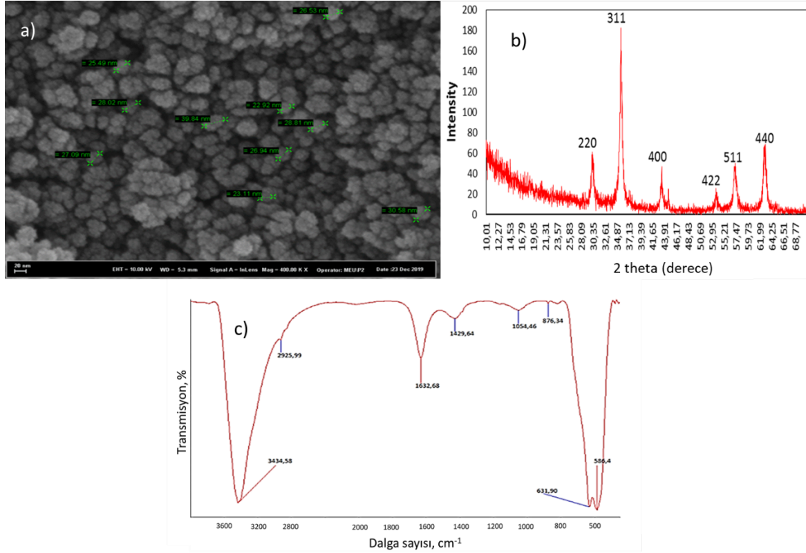
Şekil 1. Üretilen Fe 3 O 4 nanopartikül karakterizasyonu a) SEM görüntüsü, b) XRD difraktogramı, c) FTIR spektrumu
