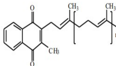
Vitamin K2
