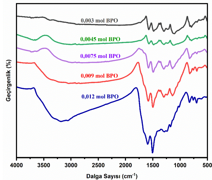
Şekil 3. Farklı BPO konsantrasyonlarındaki FT-IR spektrumları.
