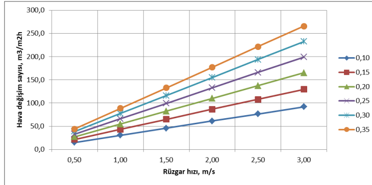
Şekil 1. Farklı havalandırma ve rüzgâr hızlarında ortaya çıkan hava değişim sayıları
