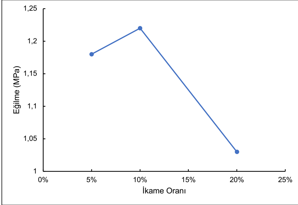
Şekil 3. 28 günlük silis proses atığı ikameli numunelerin eğilme dayanımları
