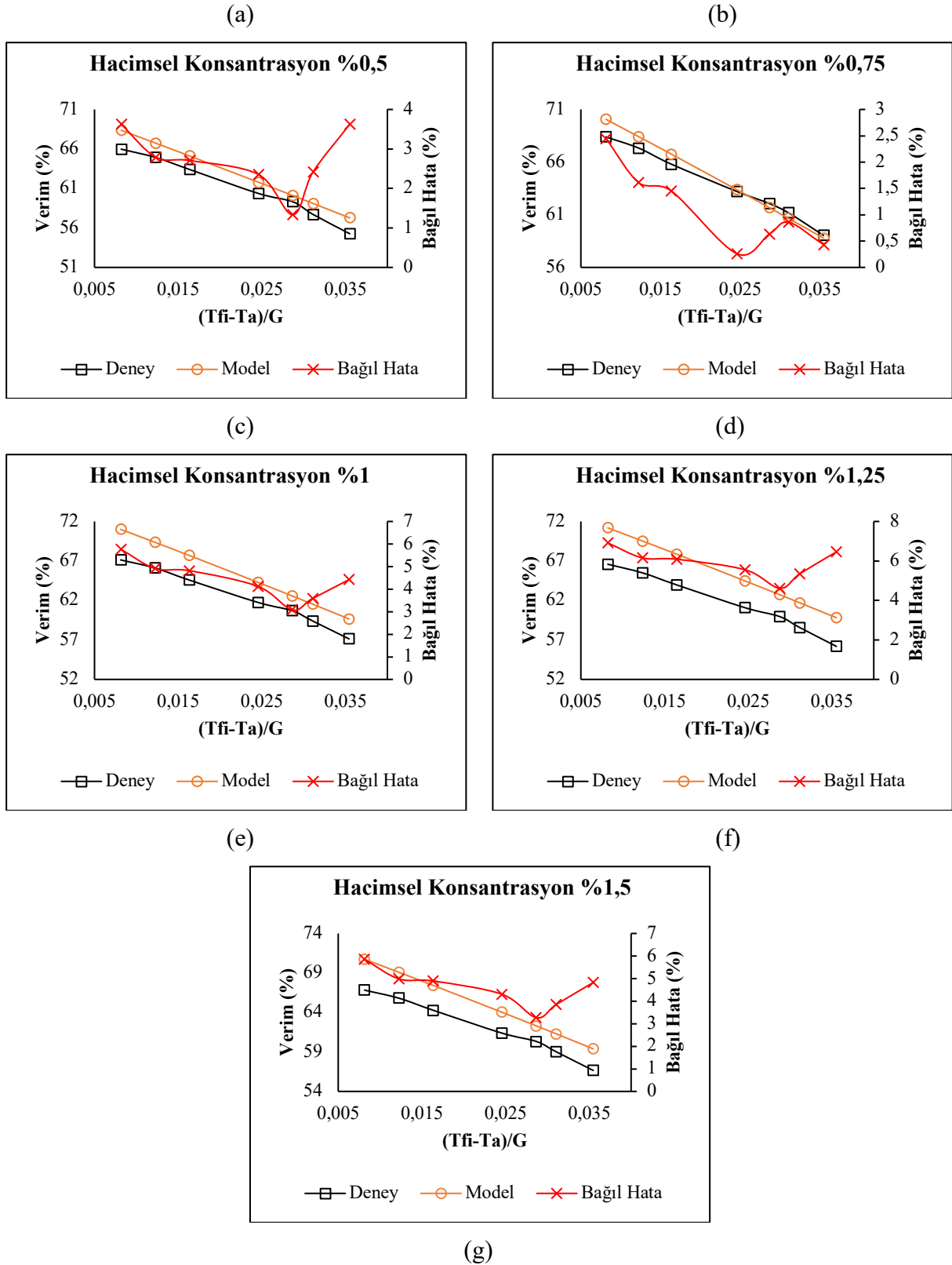
Şekil 1. MgO-su nanokışkan ile çalışan düz plakalı güneş kolektörüne ait matematiksel model ve deneysel sonuçlarının karşılaştırılması (Verma, Tiwari ve Chauhan, 2016).
