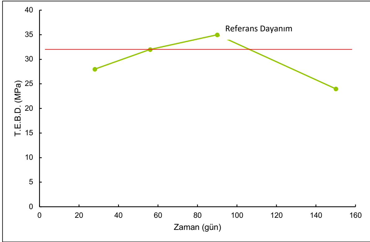
Şekil 2: %5 Altın madeni proses atığı ikamesinde zamana göre dayanım değerleri
