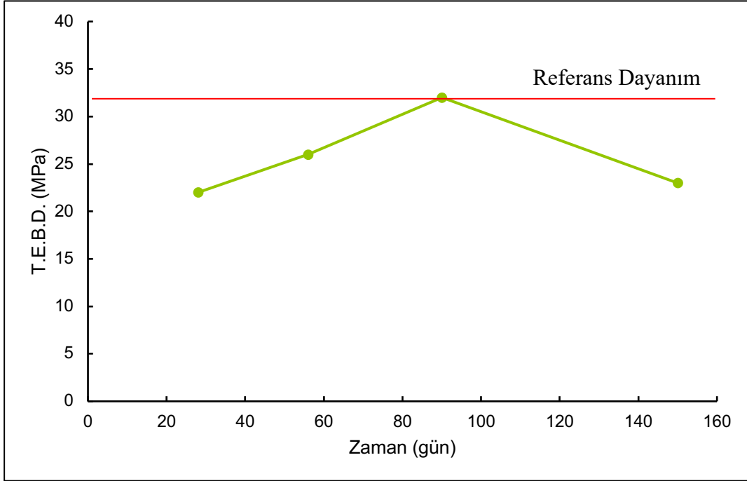
Şekil 3: %10 Altın madeni proses atığı ikamesinde zamana göre dayanım değerleri
