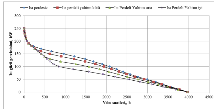
Şekil 3. Kırşehir ili iklim koşullarında ısı perdelerinin sızdırmazlıklarına bağlı olarak ortaya çıkan ısı gücü gereksinimleri
