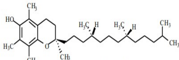
Vitamin E
