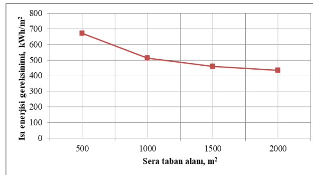
Şekil 1. Tekser ve blok olarak inşa edilen seralarda birim taban alanı için gerekli ısı enerjisi
