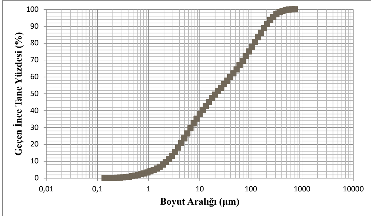
Şekil 1. Altın madeni proses atığı tane boyut dağılımı
